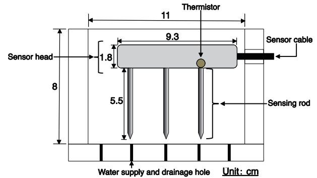
Fig. 1 実験装置図. Experimental apparatus.
