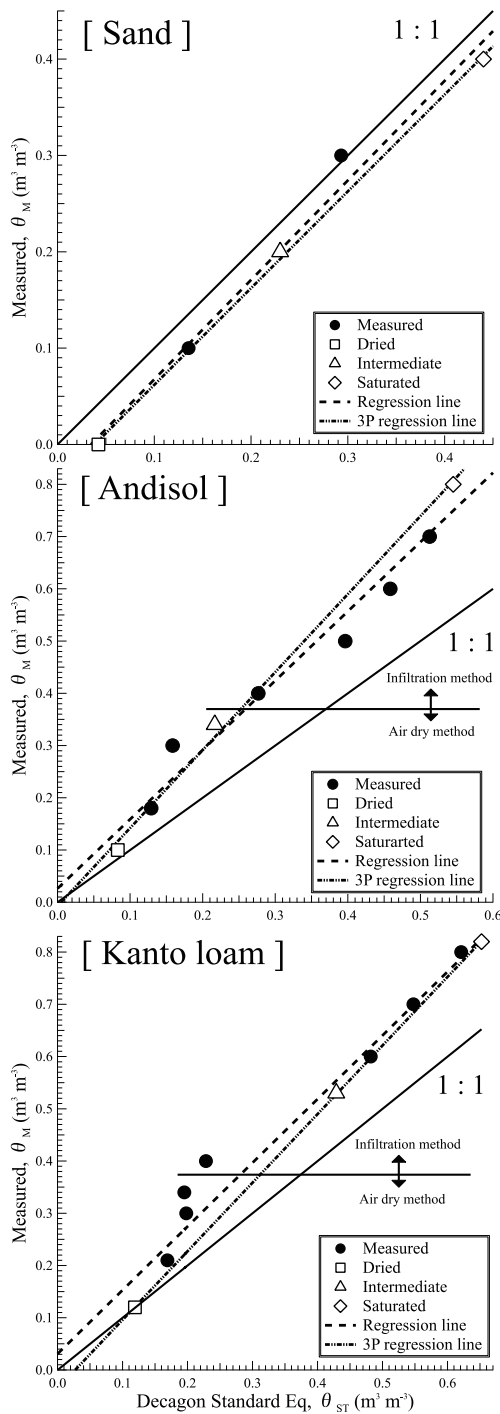
Fig. 4 3種類の土壌のGS3の標準式で求めた \theta_{ST} と重量測定に基づく \theta_M の関係(●). 実線は \theta_{ST} の1:1直線. 破線は \theta_{ST} と \theta_M の一次回帰直線. 二点鎖線は3点(乾燥:□, 中間:△, 飽和:◇)の \theta_{ST} と \theta_M から求めた一次回帰直線. 黒ボク土とローム土の図中の印は, 上下で土壌の水分調節方法(上:浸潤法, 下:風乾法)の水分領域を示す.
