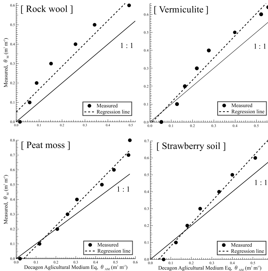
Fig. 3 4種類の農業用培地のGS3の培地式で求めた \theta_{AM} と重量測定に基づく \theta_M の関係。実線は \theta_{AM} の1:1直線。破線は \theta_{AM} と \theta_M の一次回帰直線。
