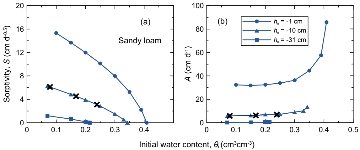
Fig. 7 異なる地表面境界圧力 h_0 に対する砂質ロームの浸潤における Philip モデルの (a) 吸水量 S と (b) 定数 A の初期水分量 \theta_i との関係。
