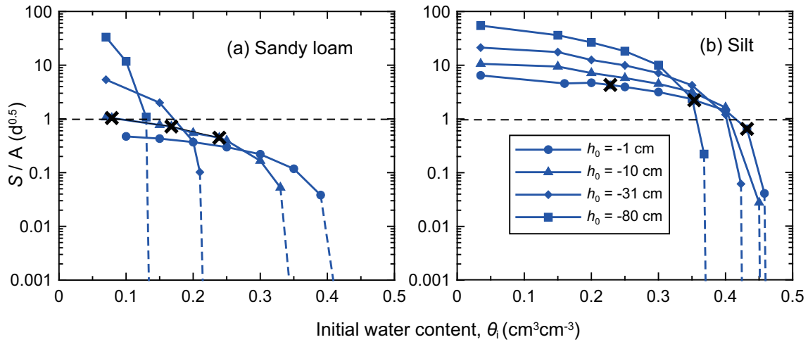
Fig. 9 異なる地表面境界圧力 h_0 に対する砂質ロームとシルトの浸潤における Philip モデルの吸湿度 S と定数 A の比 S/A と初期水分量 \theta_i との関係 (a) 砂質ローム, (b) シルト.
